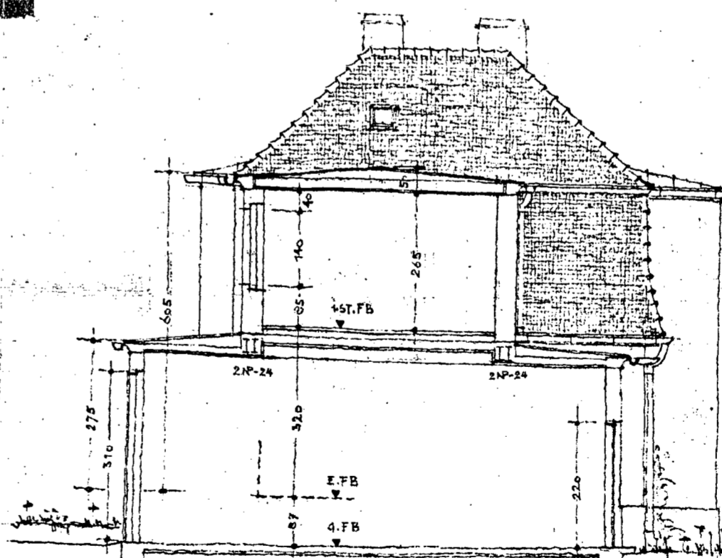
SCHNITT
