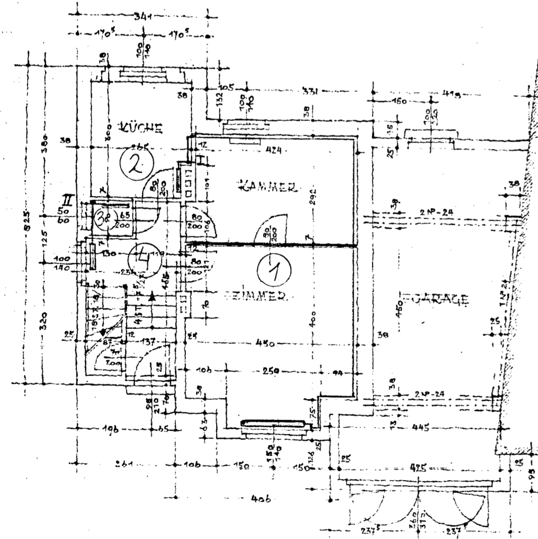
ERDGESCHOSS
