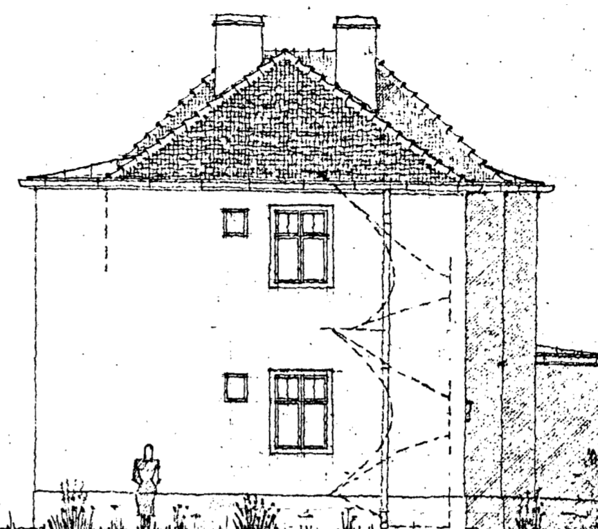
SEITENANSICHT
