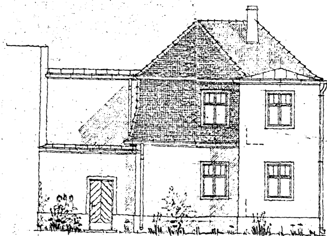
GARTENANSICHT
